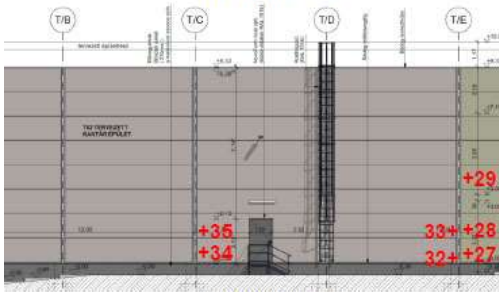
D-i homlokzat
