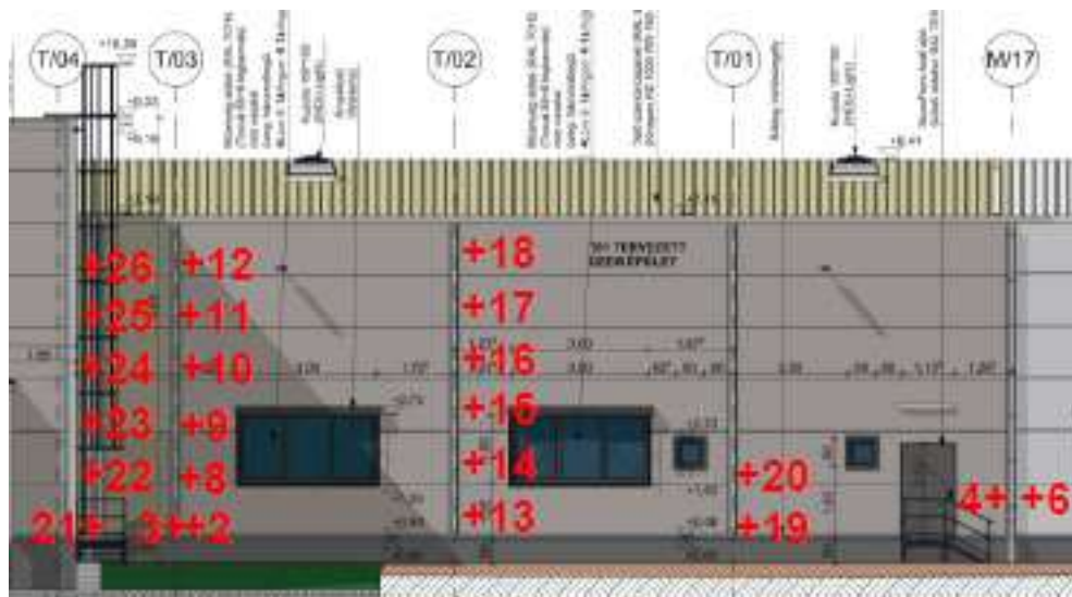
NY-i homlokzat
